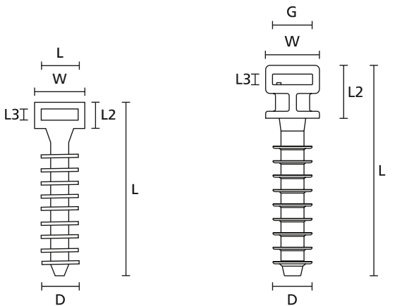
LOK01 Wanddübel (Frontansicht)
