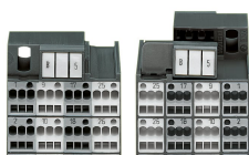
Repérage individuel du côté des réparti- tions avec le système de repérage rapide WSB
