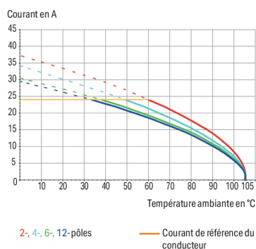
Courbe d'intensité maximale admissible Pas 5,08 mm / section de conducteur 2,5 mm 2 « s » Selon l'exemple de : EN 60512-5-2 / facteur de réduction 1
