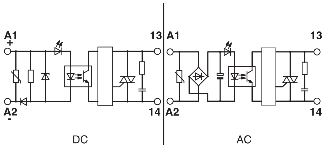
电路图
