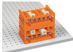
Codage d'un connecteur mâle à deux étages THT
