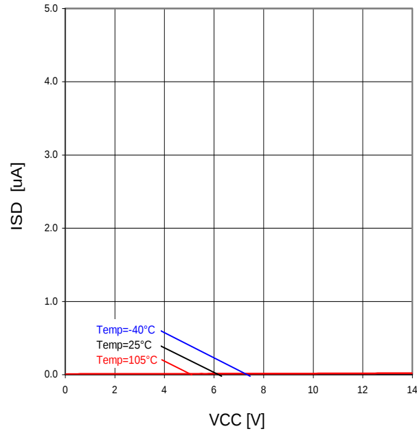
Fig.26 VCC-ISD (VEN=0V)
