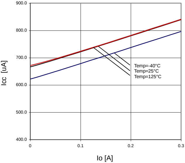
Fig.30 I_o - I_{CC}
