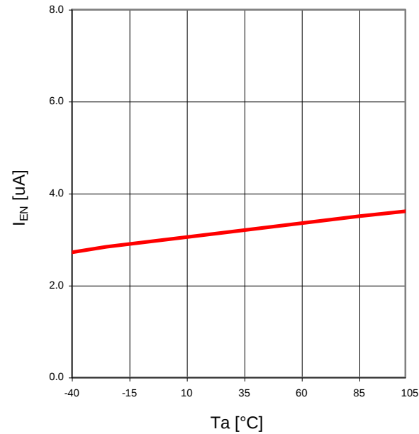
Fig.24 Ta-IEN
