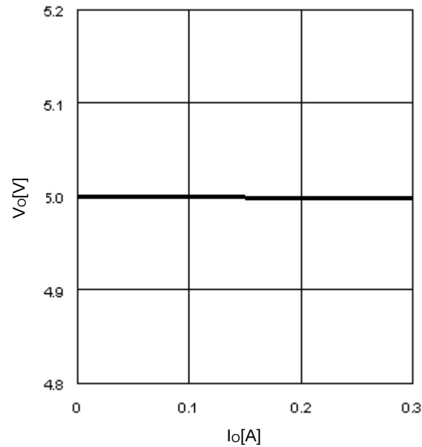
Fig.25 Io-Vo
