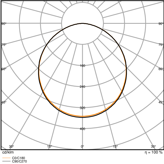
PL COMP 600 V 26W 840 3640lm
