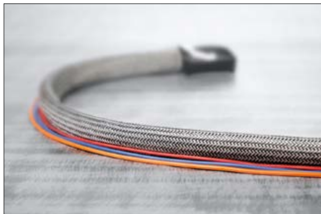
HEGEMIPV0 Geflechtschläuche: EMV-Schutz bei erhöhten Brandschutzanforderungen.
