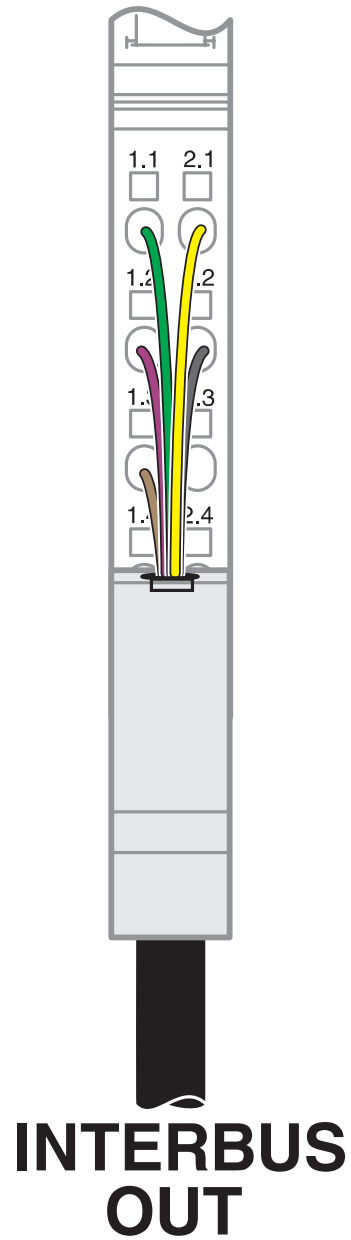
接线图
