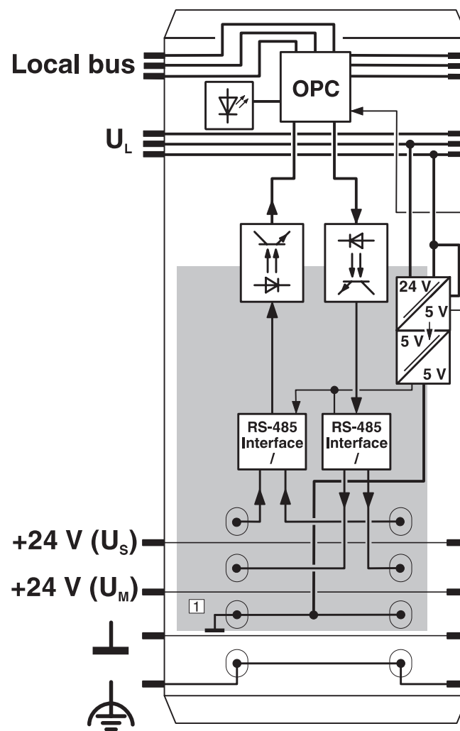
结构框图
