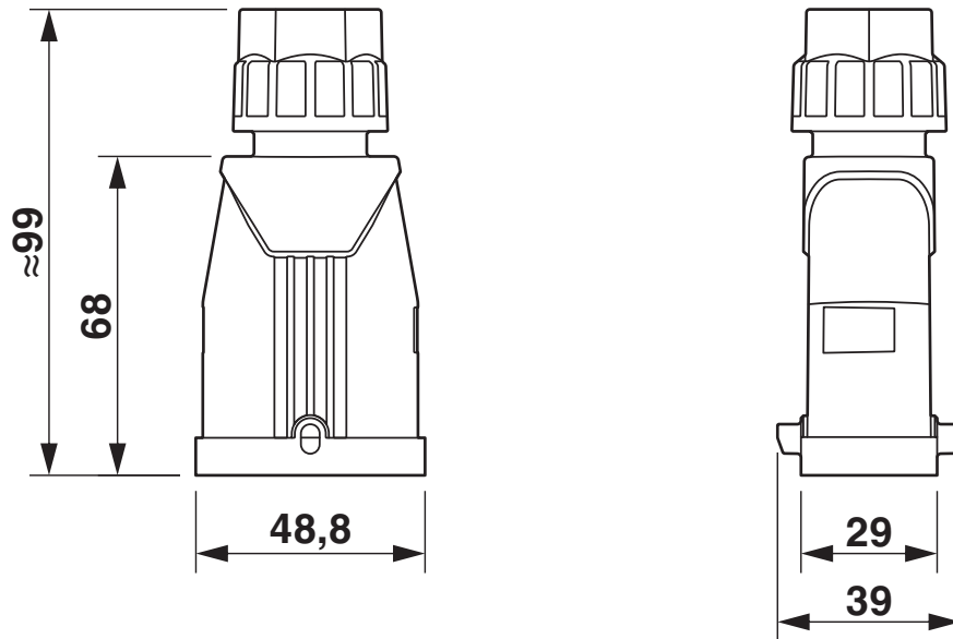
尺寸图
