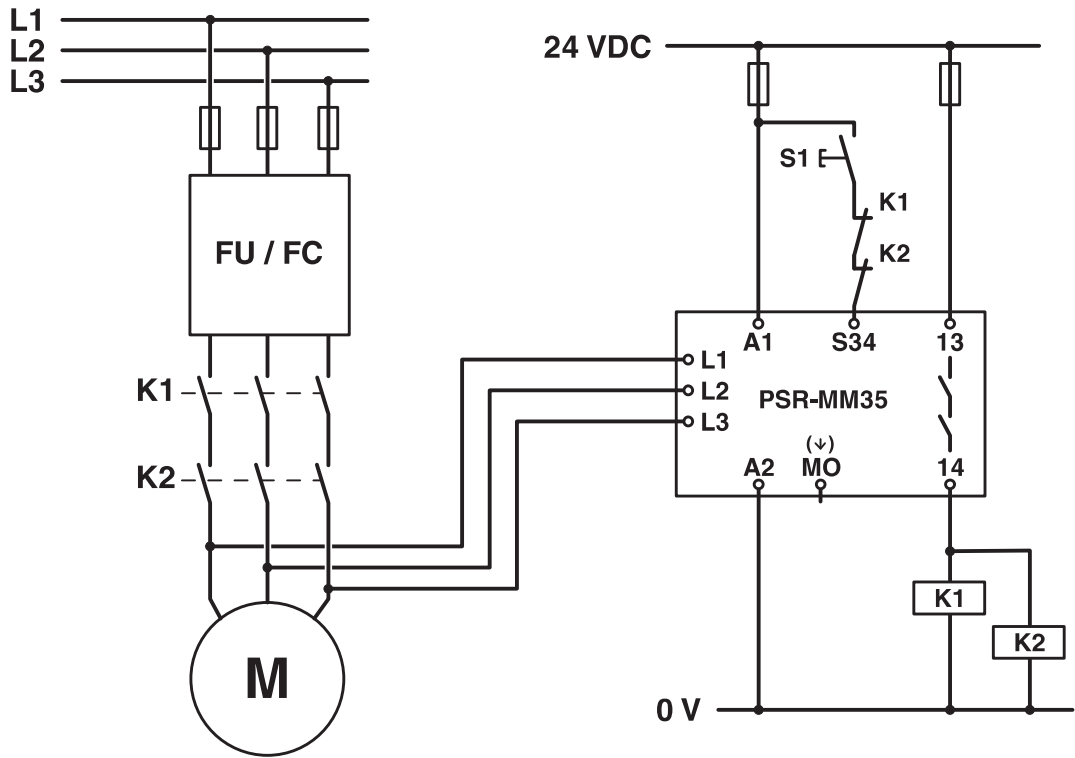
电路图
