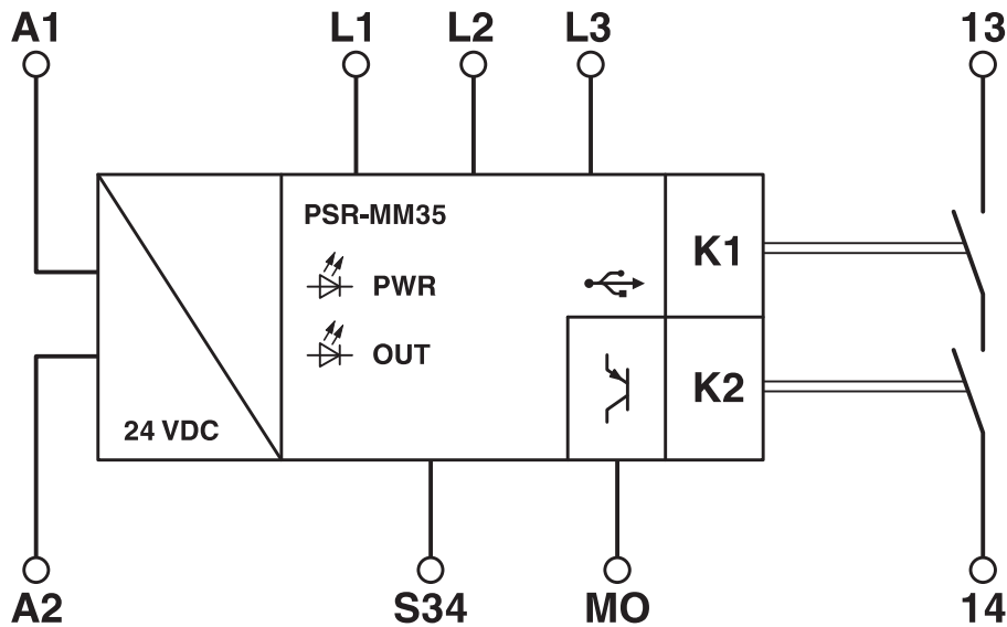
结构框图
