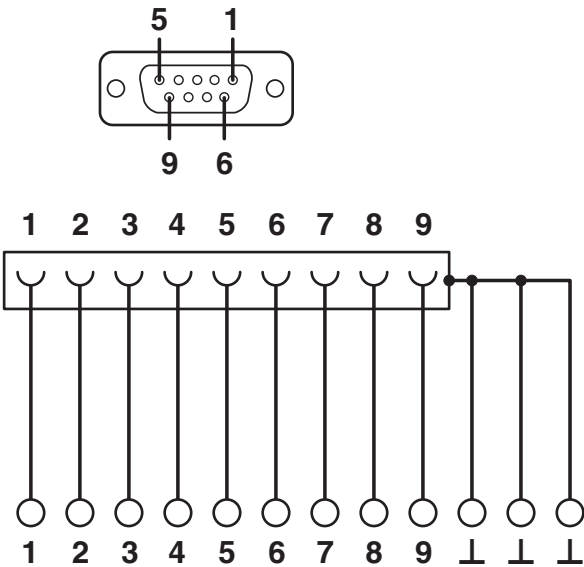
电路图
