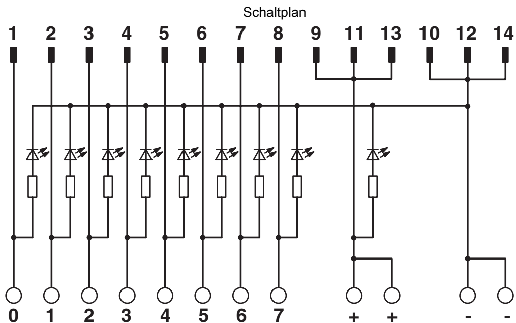
Anschlussbild VIP-2/.../FLK14/LED/PLC
