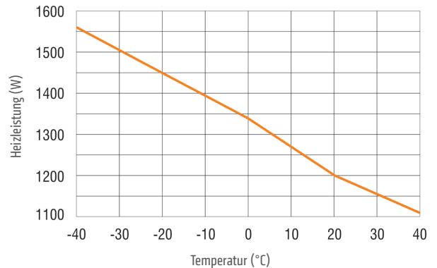
Heizleistung-/Umgebungstemperatur-Diagramm CS 030
