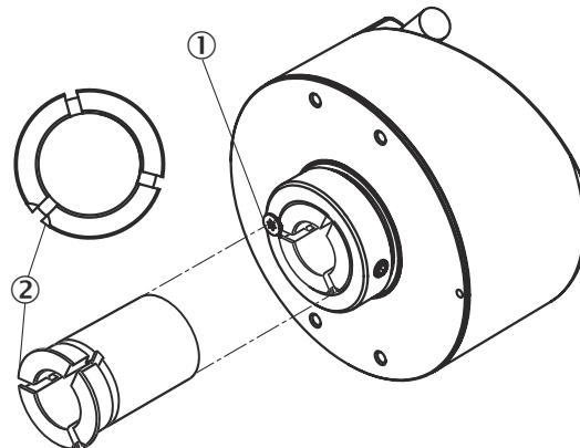
Abbildung 1: Montage Hülse für Hohlwellenencoder
