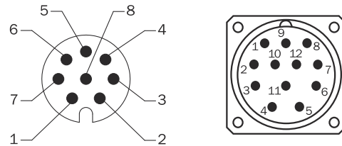
Abbildung 15: Links = Ansicht Gerätestecker M12 Rechts = Ansicht Gerätestecker M23
