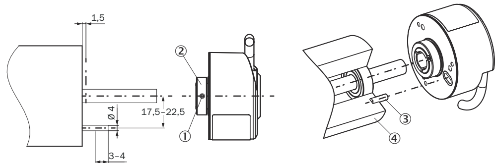
Abbildung 6: Anbau mit axialer Passstiftmontage Variante K
