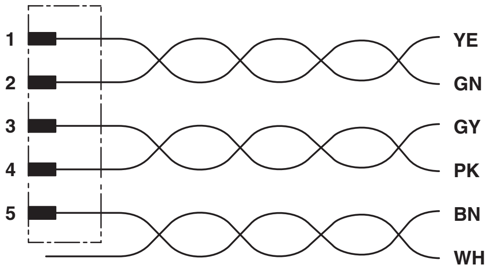
电路图
