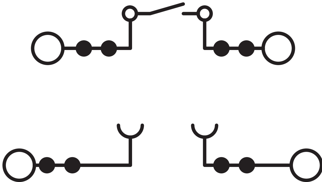
电路图
