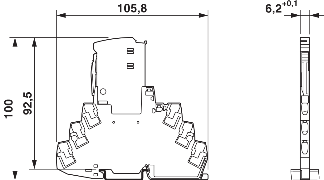
尺寸图
