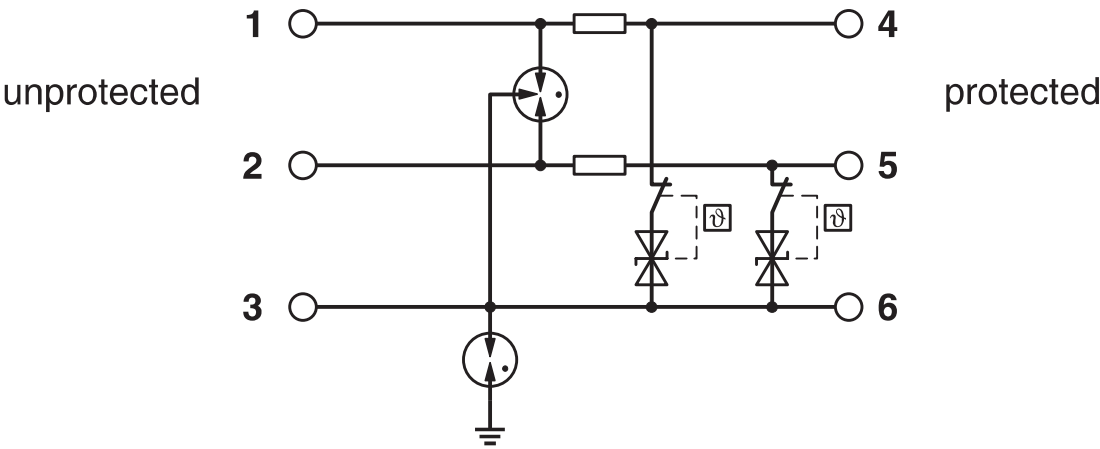
电路图
