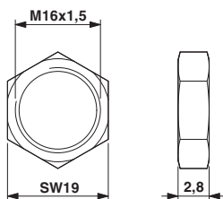
Disegno quotato
