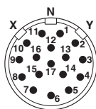
配線図
