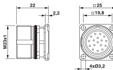
外形寸法
