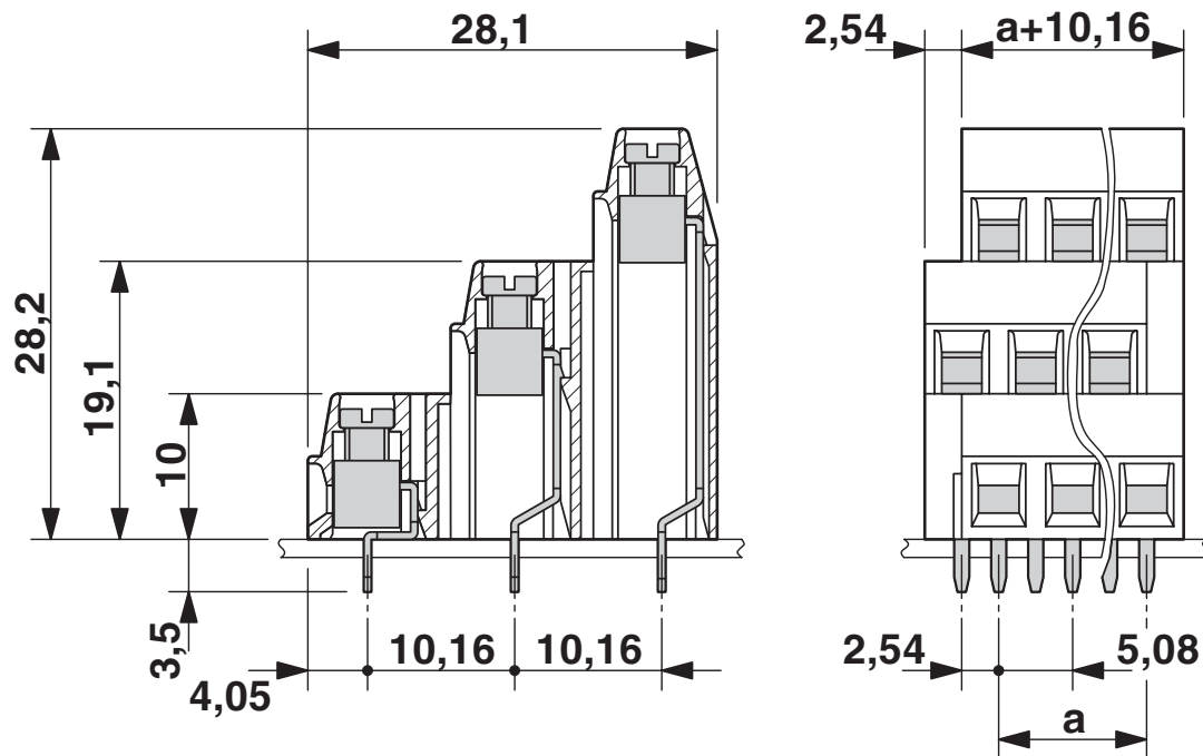
尺寸图
