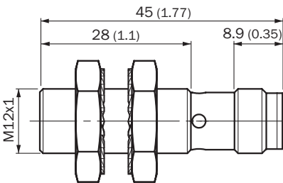
IMB12 短版, M12 插头, 齐平
