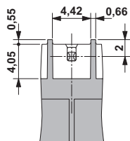
外形寸法
