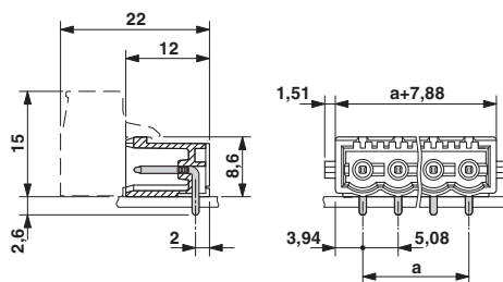
外形寸法
