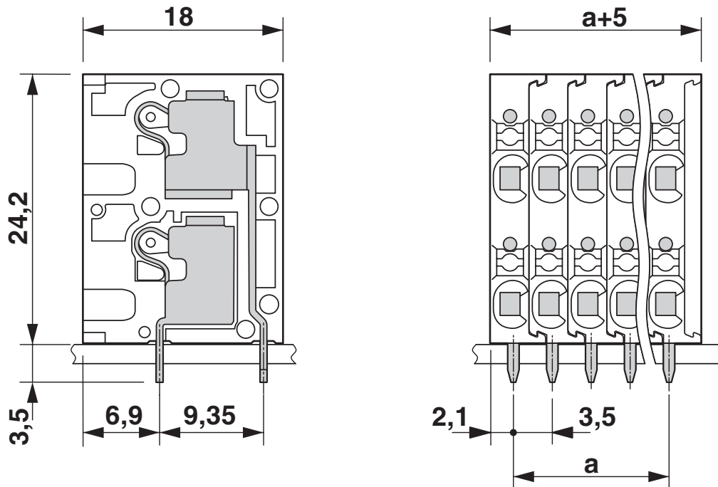
尺寸图
