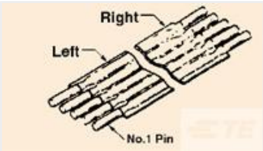
TE Part #7-1437212-4 FSK-22A-6
