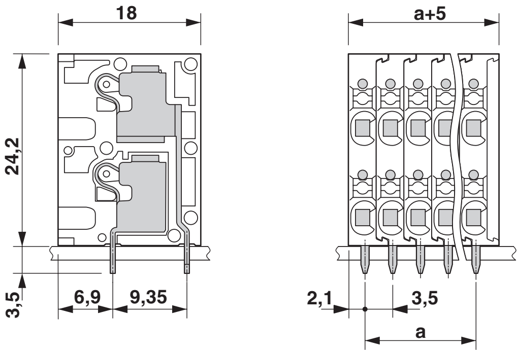
尺寸图
