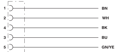
M12ソケットのコンタクトアサイン
