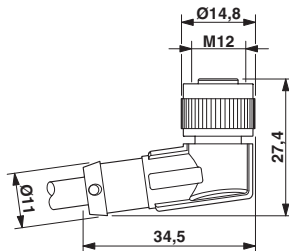
外形寸法
