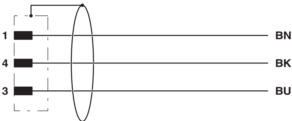
电路图
