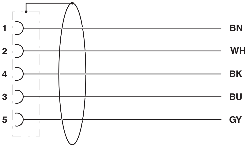
电路图
