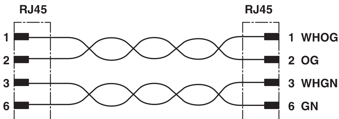
电路图
