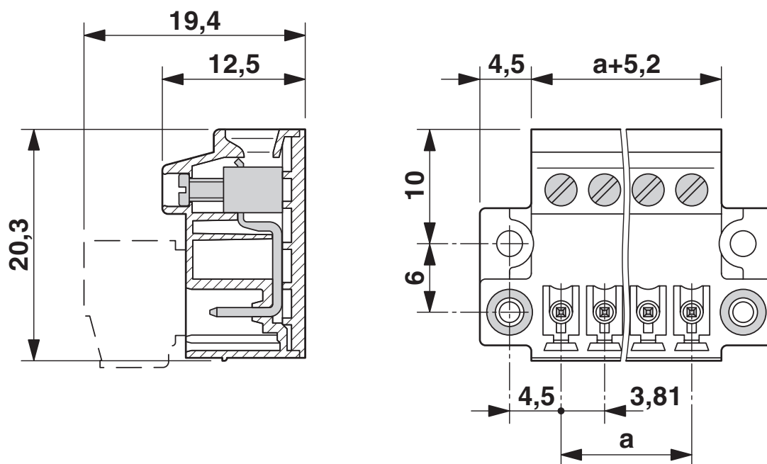
尺寸图
