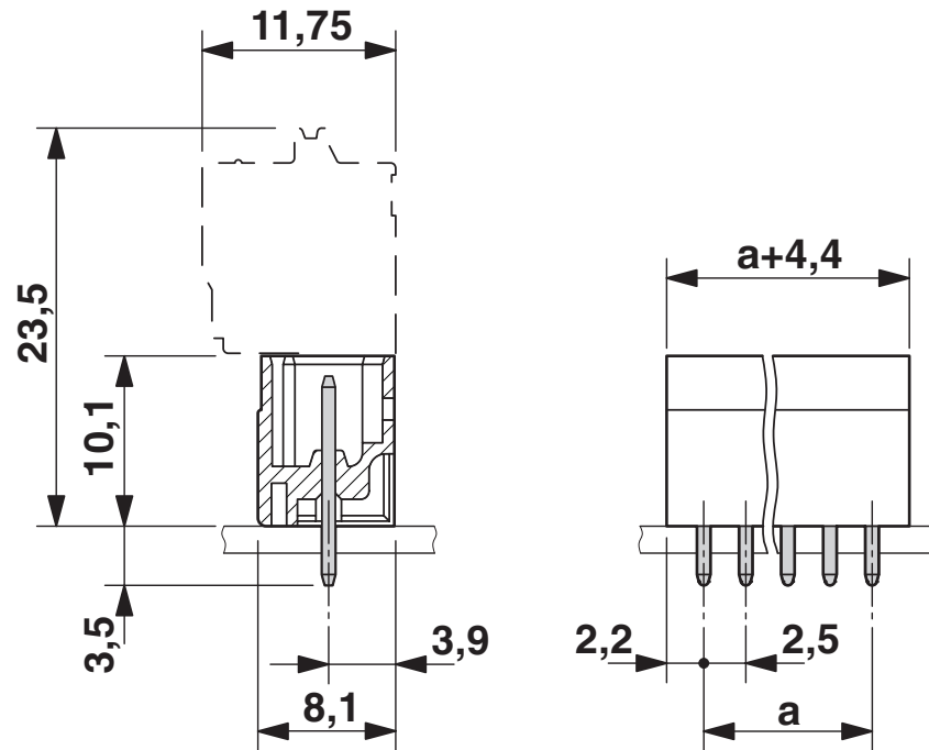
尺寸图
