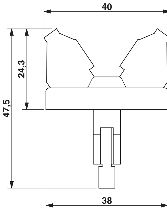
Maßzeichnung
