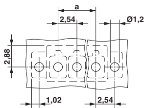
穴あけ加工図
