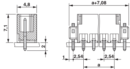
外形寸法
