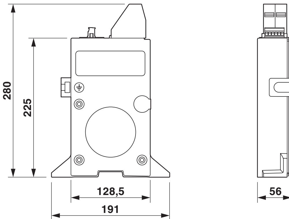
尺寸图
