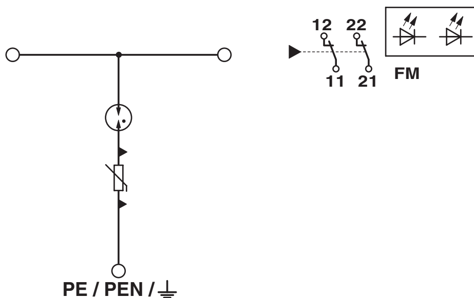
电路图
