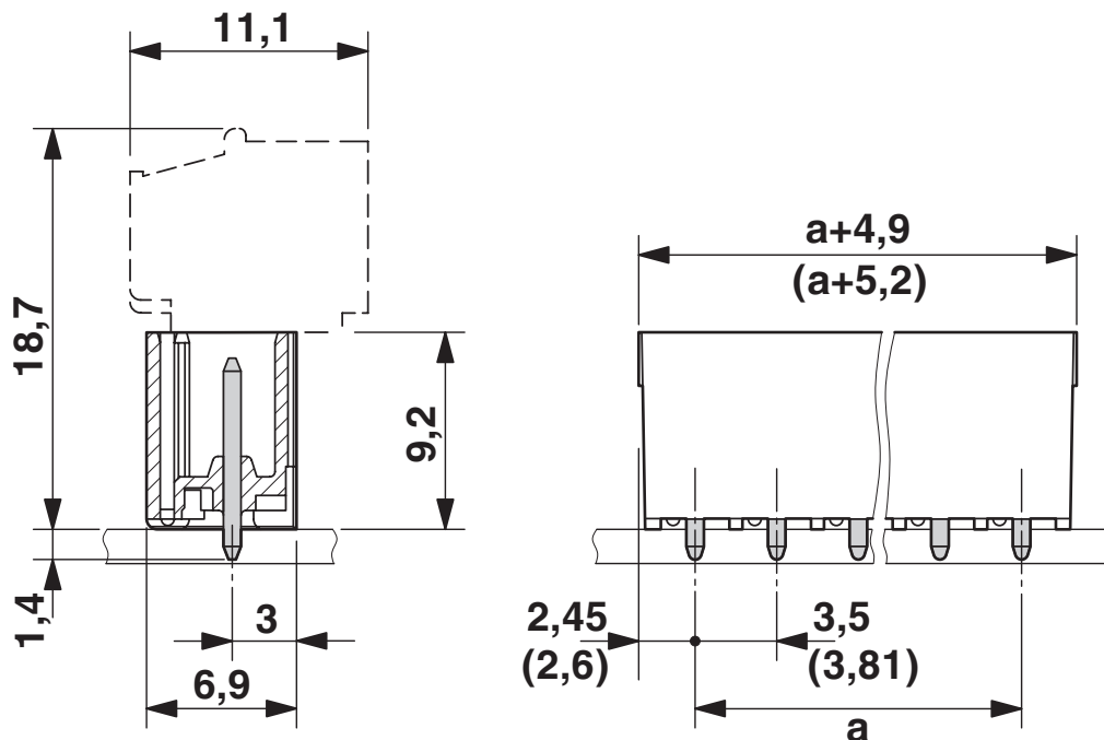
Maßzeichnung
