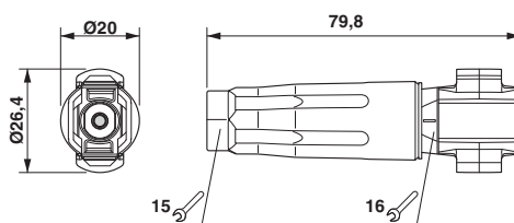
Dessin coté
