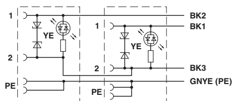
回路図
