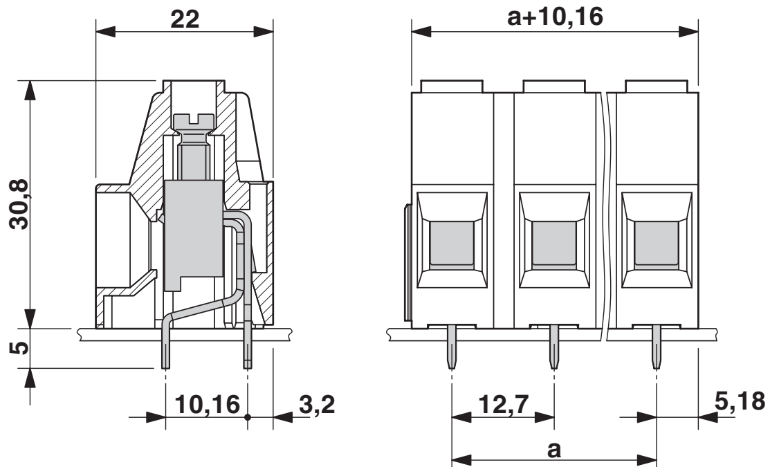
尺寸图
