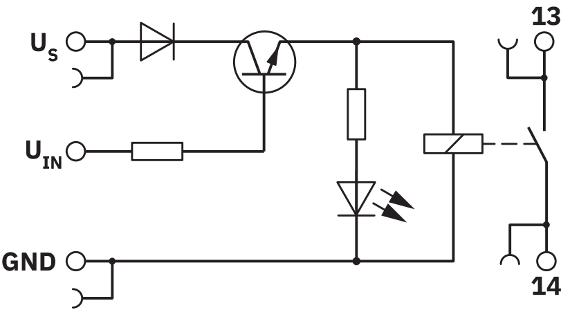
电路图
