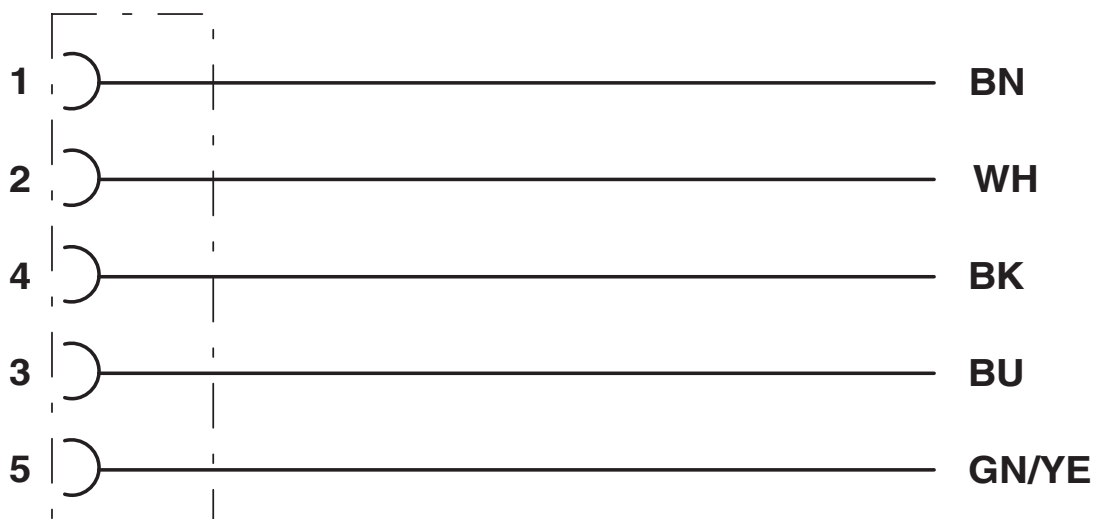
电路图
