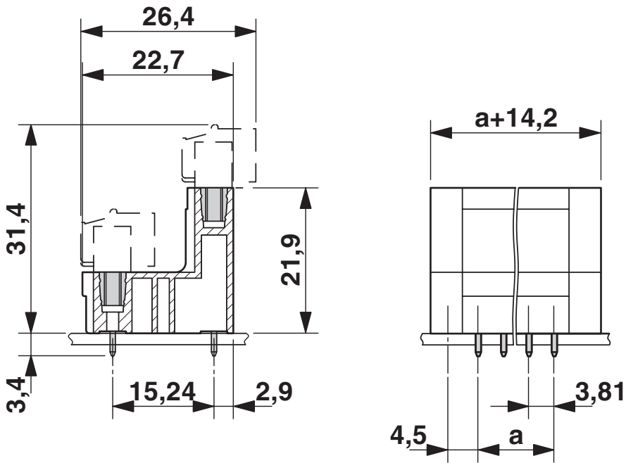
尺寸图
