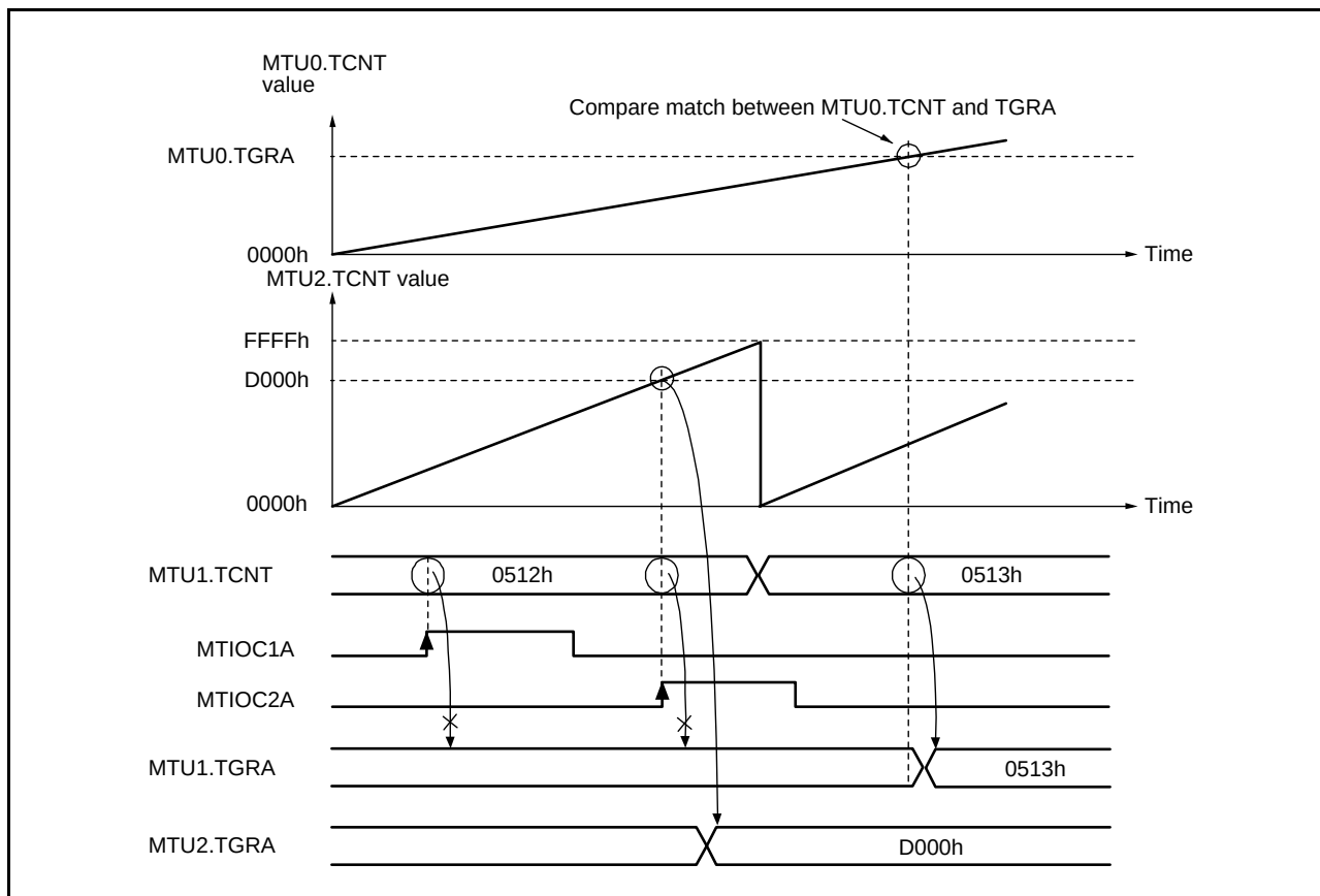
Figure 22.24 Cascaded Operation Example (d)
