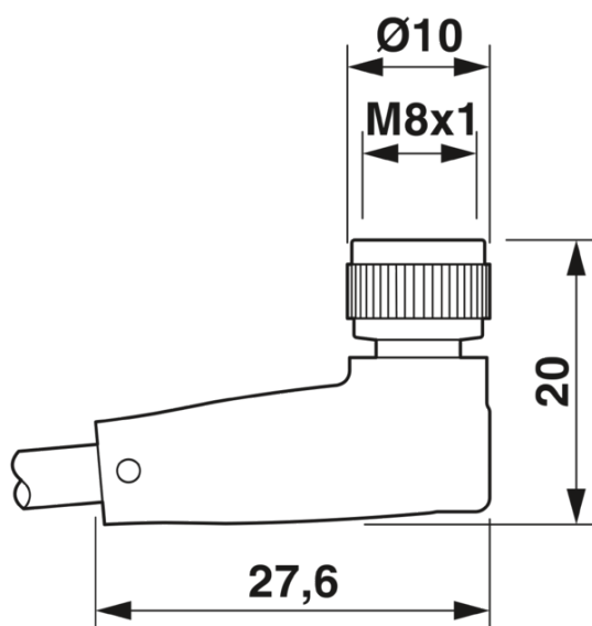
Rysunek wymiarowy
