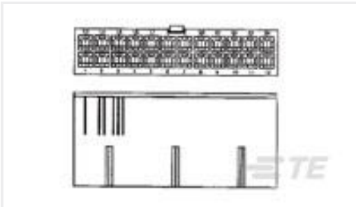
TE Part #1586000-2 2P FH PLUG VAL-U-LOK V2
