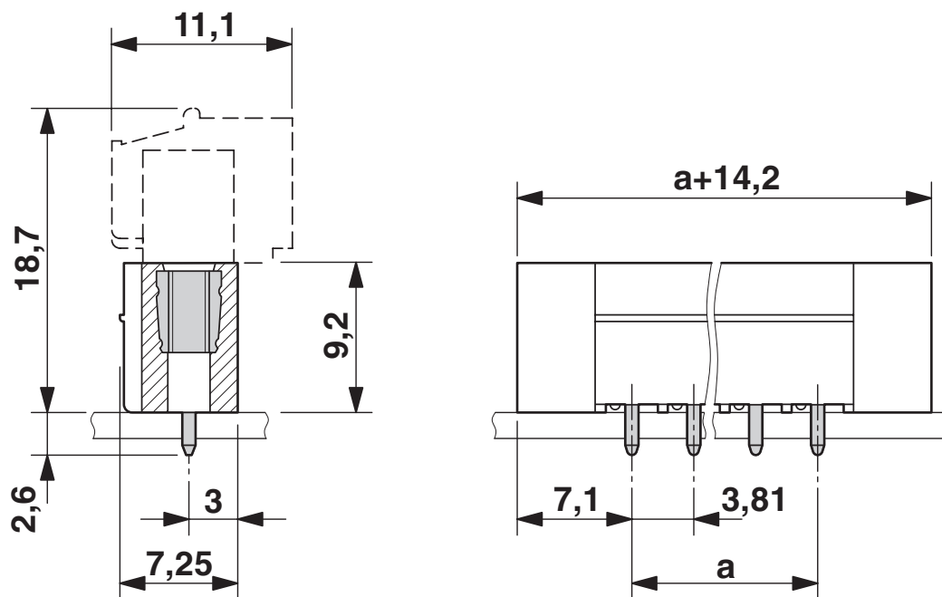
尺寸图
