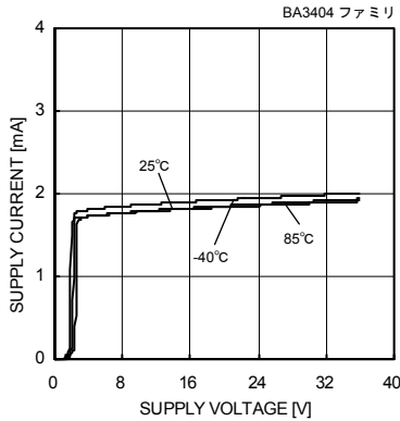
Fig. 98 回路電流－電源電圧特性
