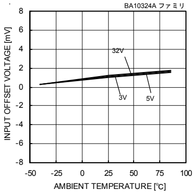
Fig. 37 入力オフセット電圧－温度特性 (Vicm=0[V], VOUT=1.4[V])
