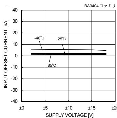
Fig. 107 入力オフセット電流－電源電圧特性 (Vicm=0[V], VOUT=0[V])
