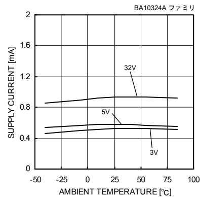
Fig. 27 回路電流－温度特性
