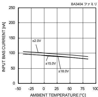
Fig. 106 入力バイアス電流－温度特性 (Vicm=0[V], VOUT=0[V])
