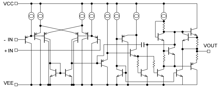
Fig. 120 内部等価回路図 (BA3404)
