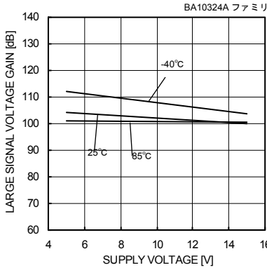
Fig. 44 大振幅電圧利得－電源電圧特性 (RL=2[kΩ])
