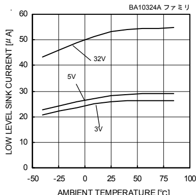
Fig. 35 LOW レベルシンク電流－温度特性 ( V_{OUT}=0.2[V] )
