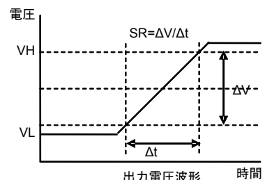
Fig. 123 スルーレート測定時 入出力波形例
