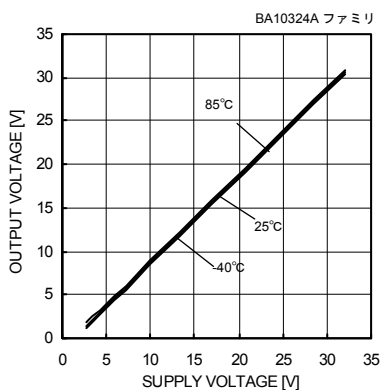
Fig. 28 出力電圧－電源電圧特性 ( R_L=10[k\Omega] )
