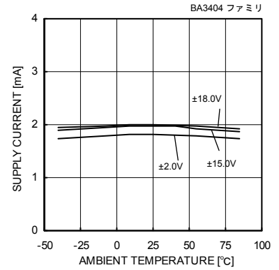
Fig. 99 回路電流－温度特性
