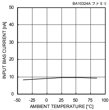
Fig. 40 入力バイアス電流－温度特性 (VCC=30[V], Vicm=28[V], VOUT=1.4[V])
