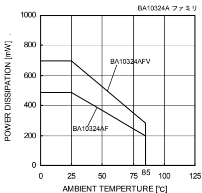
Fig. 25 ディレーティングカーブ
