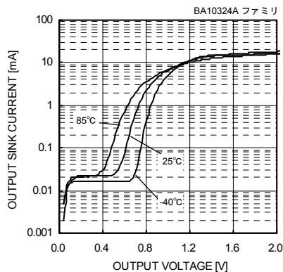
Fig. 32 出力シンク電流－出力電圧特性 ( V_{CC}=5[V] )
