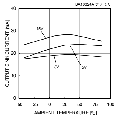
Fig. 33 出力シンク電流－温度特性 ( V_{OUT}=V_{CC} )
