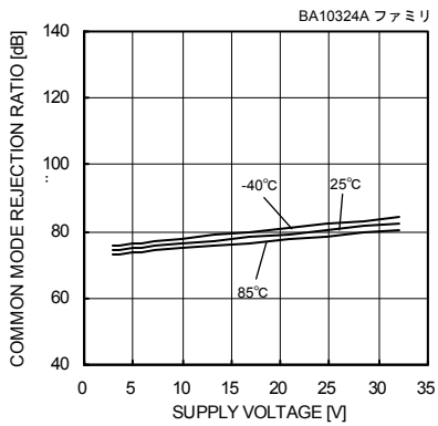
Fig. 46 同相信号除去比－電源電圧特性
