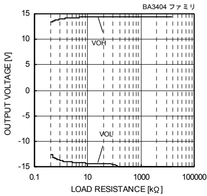
Fig. 100 出力電圧－負荷抵抗特性 (VCC/VEE=+15[V]/-15[V], Ta=25[°C])
