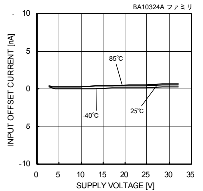
Fig. 42 入力オフセット電流－電源電圧特性 (Vicm=0[V], VOUT=1.4[V])
