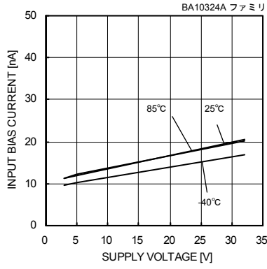
Fig. 38 入力バイアス電流－電源電圧特性 (Vicm=0[V], VOUT=1.4[V])
