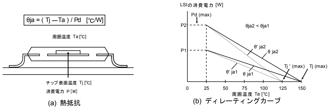
Fig. 125 熱抵抗とディレーティングカーブ
