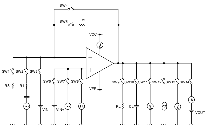
Fig.122 測定回路例2 (片チャンネルのみ)
