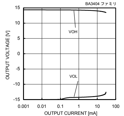
Fig. 102 出力電圧－出力電流特性 (VCC/VEE=+15[V]/-15[V], Ta=25[°C])
