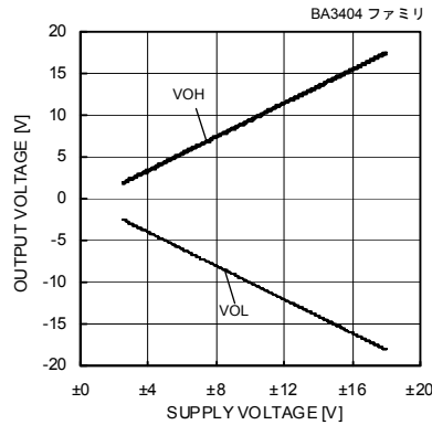
Fig. 101 最大出力電圧－電源電圧特性
