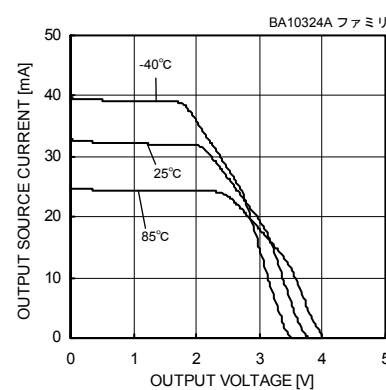
Fig. 30 出力ソース電流－出力電圧特性 ( V_{CC}=5[V] )
