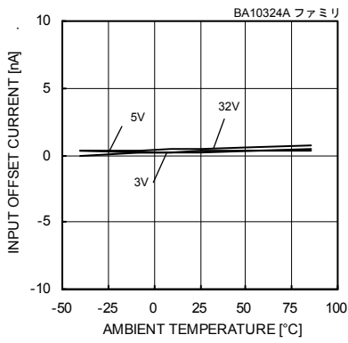
Fig. 43 入力オフセット電流－温度特性 (Vicm=0[V], VOUT=1.4[V])
