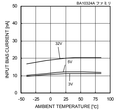
Fig. 39 入力バイアス電流－温度特性 (Vicm=0[V], VOUT=1.4[V])
