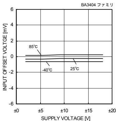
Fig. 103 入力オフセット電圧－電源電圧特性 (Vicm=0[V], VOUT=0[V])
