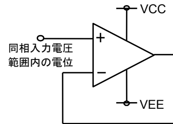
Fig. 127 未使用回路の処理例
