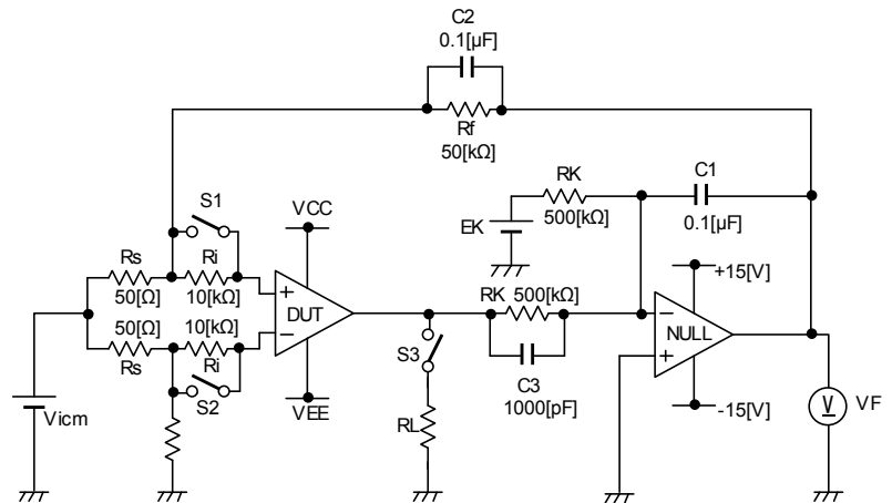
Fig. 121 測定回路例 1 (1チャンネルのみ)
