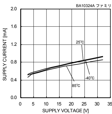
Fig. 26 回路電流－電源電圧特性
