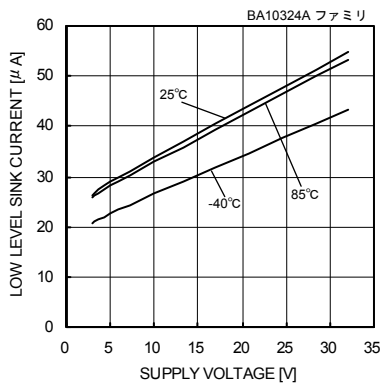
Fig. 34 LOW レベルシンク電流－電源電圧特性 ( V_{OUT}=0.2[V] )
