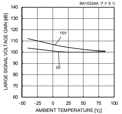
Fig. 45 大振幅電圧利得－温度特性 (RL=2[kΩ])
