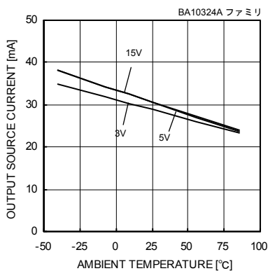
Fig. 31 出力ソース電流－温度特性 ( V_{OUT}=0[V] )
