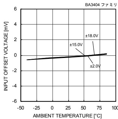
Fig. 104 入力オフセット電圧－温度特性 (Vicm=0[V], VOUT=0[V])
