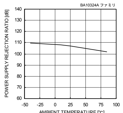
Fig. 48 電源電圧除去比－温度特性
