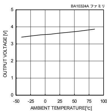
Fig. 29 最大出力電圧－温度特性 ( V_{CC}=5[V] , R_L=2[k\Omega] )
