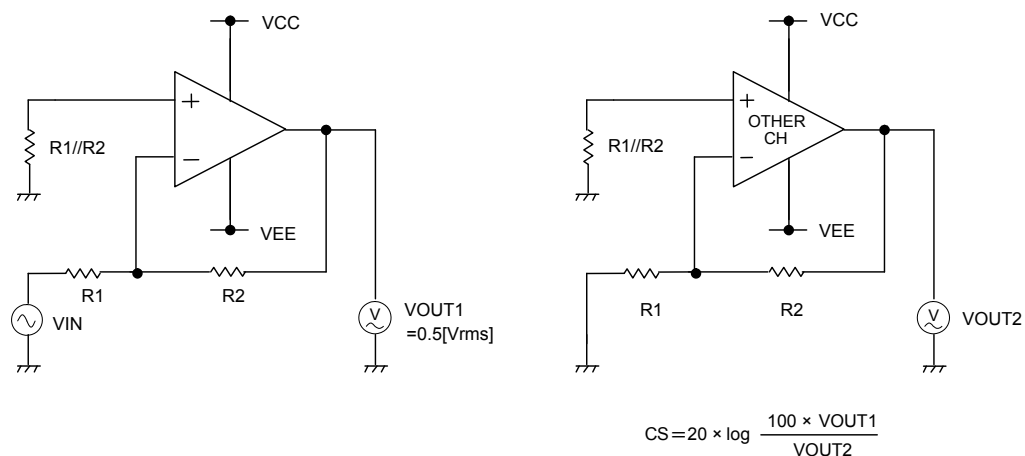
Fig. 124 測定回路例3
