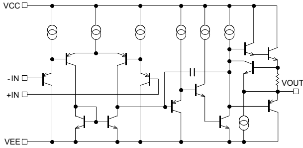
Fig. 119 内部等価回路図 (BA10358/BA10324A/BA2904S/ BA2904/BA2902S/BA2902)
