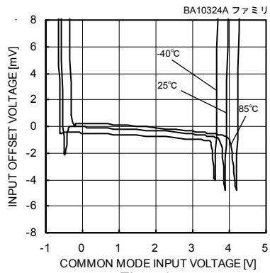
Fig. 41 入力オフセット電圧－同相入力電圧特性 (VCC=5[V])
