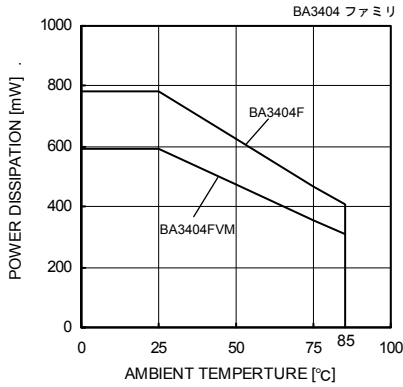
Fig. 97 ディレーティングカーブ
