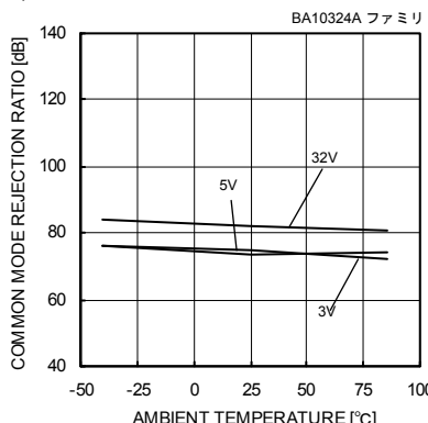
Fig. 47 同相信号除去比－温度特性
