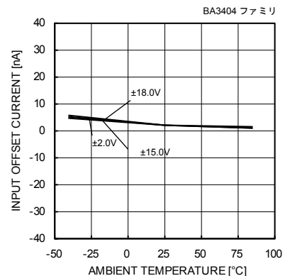
Fig. 108 入力オフセット電流－温度特性 (Vicm=0[V], VOUT=0[V])
