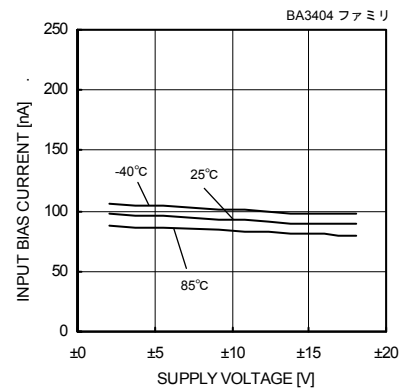
Fig. 105 入力バイアス電流－電源電圧特性 (Vicm=0[V], VOUT=0[V])
