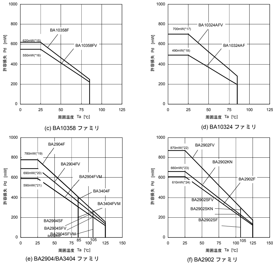
Fig. 125 熱抵抗とディレーティングカーブ
