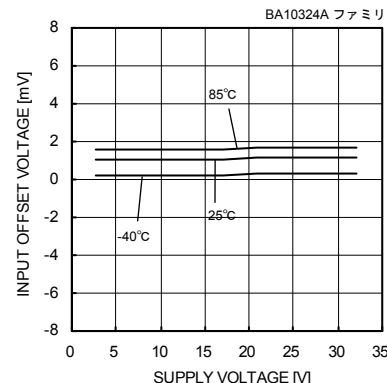
Fig. 36 入力オフセット電圧－電源電圧特性 ( V_{icm}=0[V] , V_{OUT}=1.4[V] )
