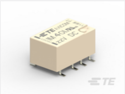
TE Part #1462047-7 IM40IGR=IM RELAY 100mW 1.5V BIS
