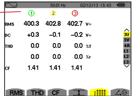
Figura 67: Lo schermo di visualizzazione simultanea in 3U
