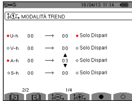
Figura 33: Il secondo schermo del modo tendenza in corso di modifica
