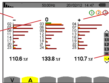
Figura 51: Lo schermo del modo esperto per la corrente
