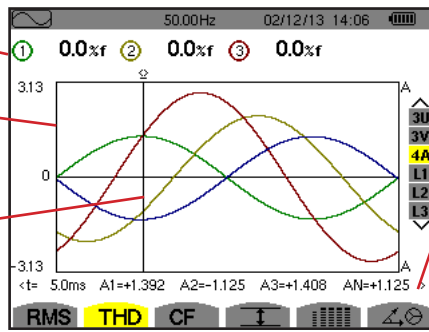
Figura 59: Lo schermo di visualizzazione THD in 4A
