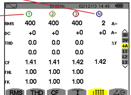
Figura 69: Lo schermo di visualizzazione simultanea in 4A
