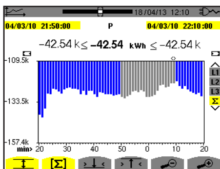
Figura 90: Ph ( \Sigma ) con MIN-AVG-MAX
