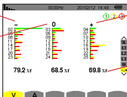
Figura 50: Lo schermo del modo esperto per la tensione semplice (montaggi trifasi con neutro)
