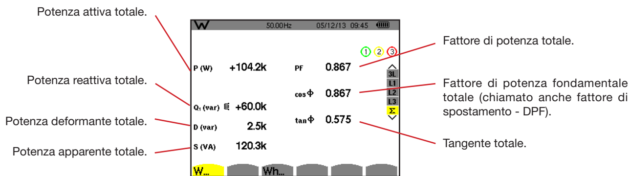
Figura 103: Lo schermo di visualizzazione delle potenze e delle grandezze totali associate in \Sigma
