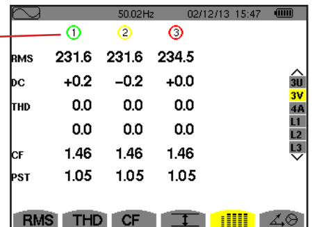
Figura 68: Lo schermo di visualizzazione simultanea in 3V
