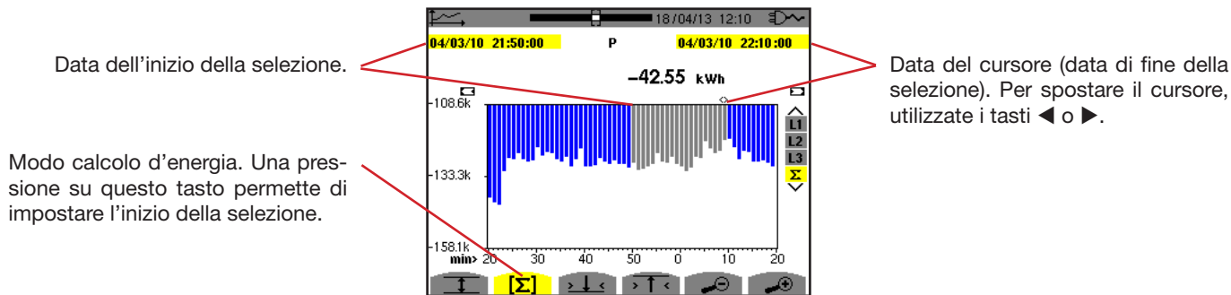
Figura 89: Ph ( \Sigma ) senza MIN-AVG-MAX
