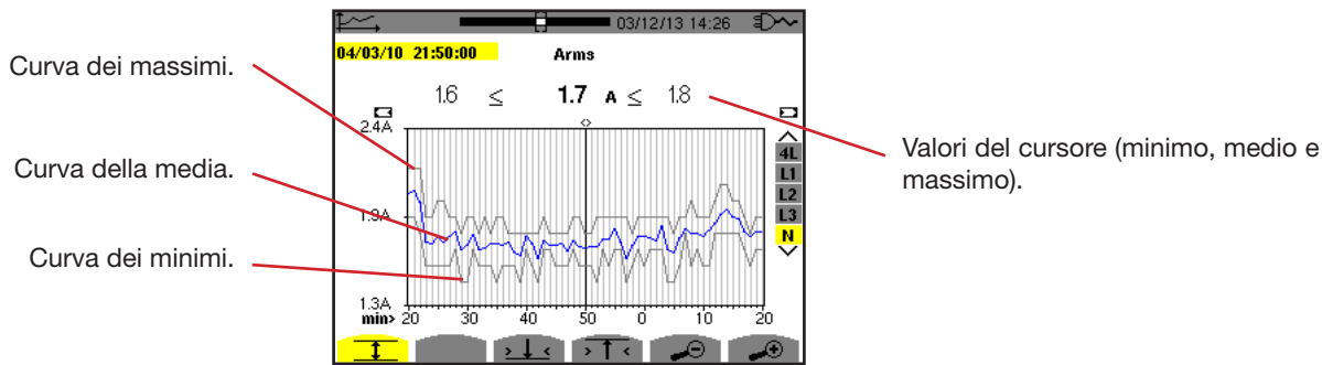
Figura 82: Arms (N) con MIN-AVG-MAX
