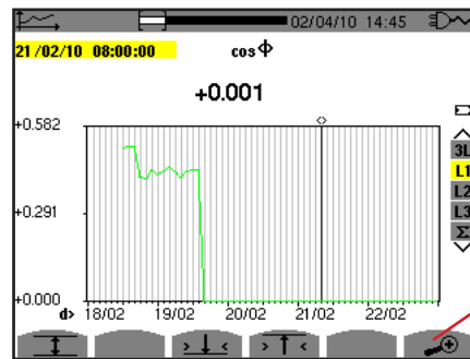
Figura 95: cos Φ (L1) caricamento / calcolo dei valori completo senza MIN-AVG-MAX per un collegamento trifase con neutro.
