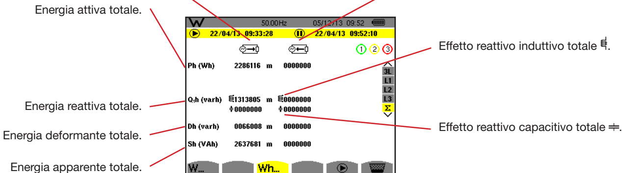
Figura 104: Lo schermo di visualizzazione delle energie consumate e generate totali in \Sigma
