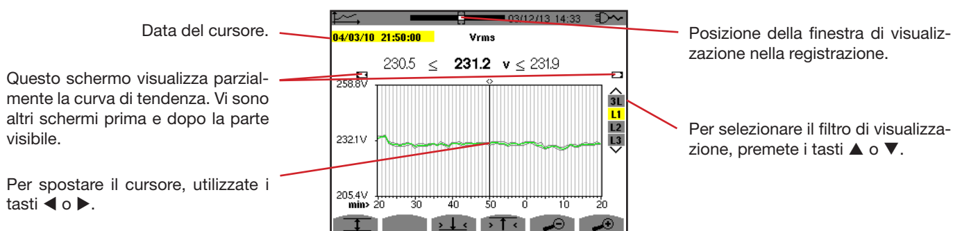
Figura 83: Vrms (L1) senza MIN-AVG-MAX
