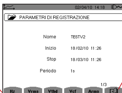
Figura 78: Lo schermo caratteristiche della registrazione
