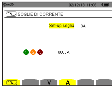
Figura 30: Lo schermo Soglie di corrente nel menu Modo transitorio
