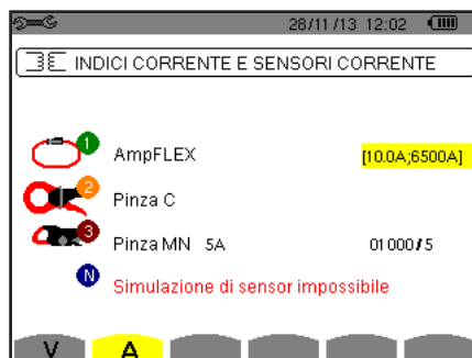
Figura 26: Lo schermo Sensori e indici di corrente nel menu Sensori e indici
