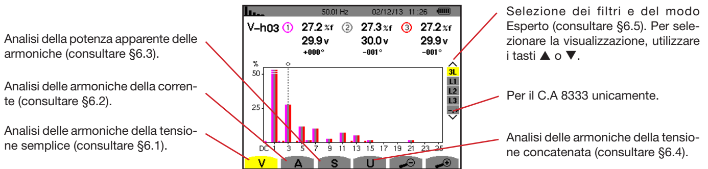
Figura 41: Lo schermo del modo armoniche
