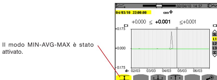
Figura 92: \cos \Phi (L1) con MIN-AVG-MAX
