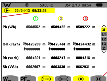
Figura 105: Lo schermo d'avviamento del conteggio d'energia in Wh
