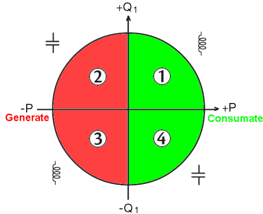
Figura 111: Diagramma dei 4 quadranti
