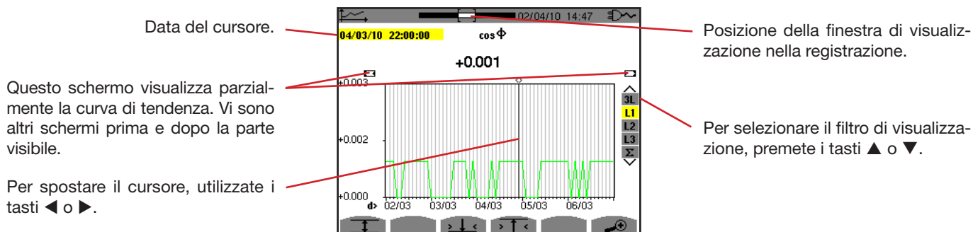
Figura 91: \cos \Phi (L1) senza MIN-AVG-MAX
