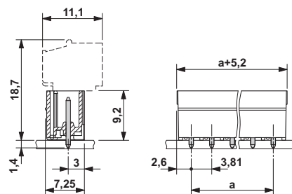
外形寸法
